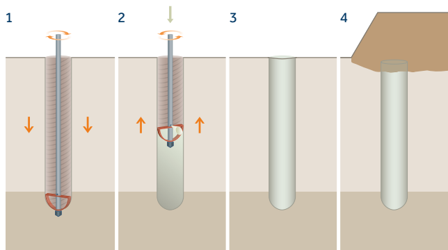
Het droog-mengsysteem
